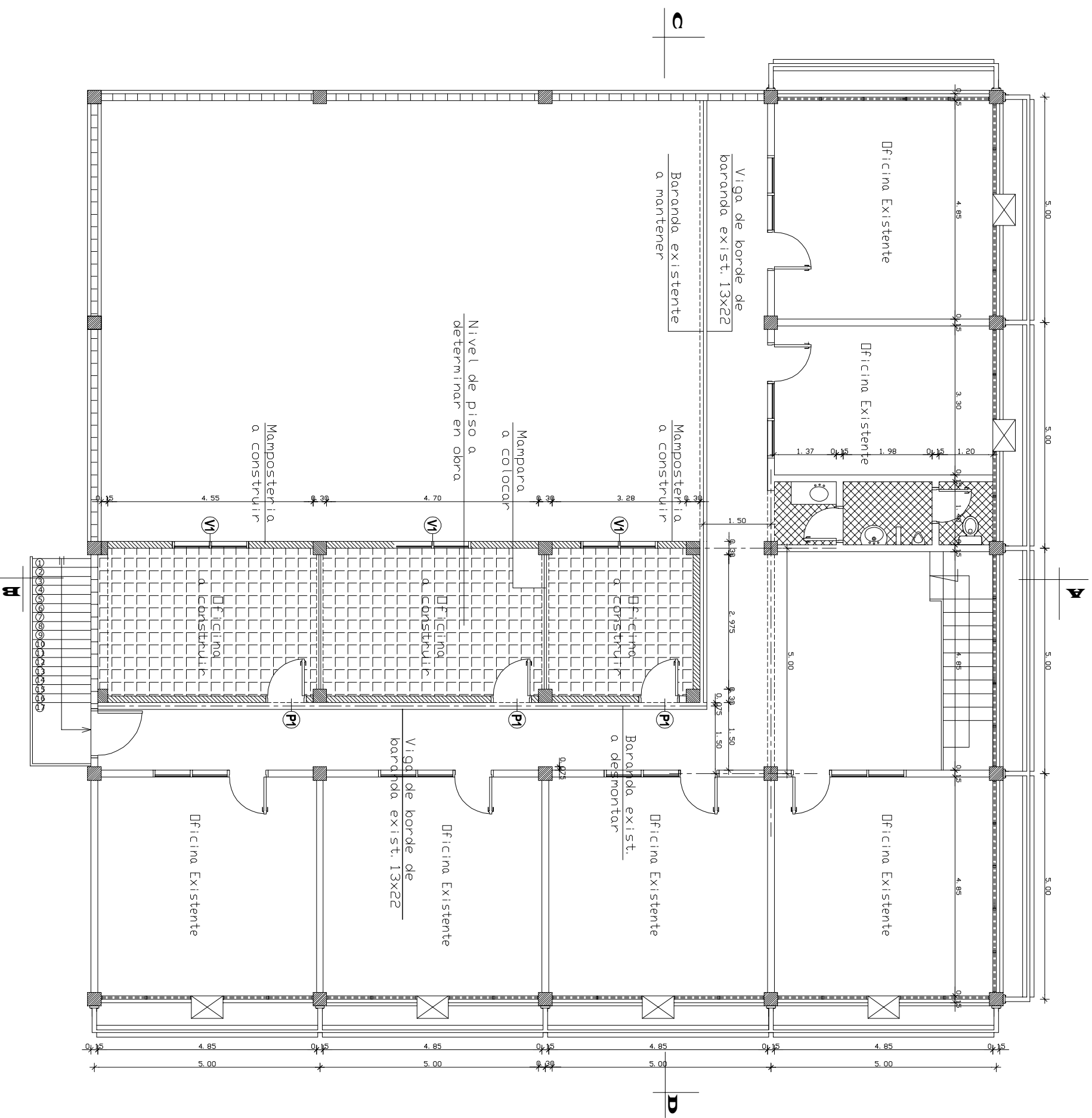
PLANTA ALTA EDIFICIO CENTRO TECNICO Esc.: .....1:100
