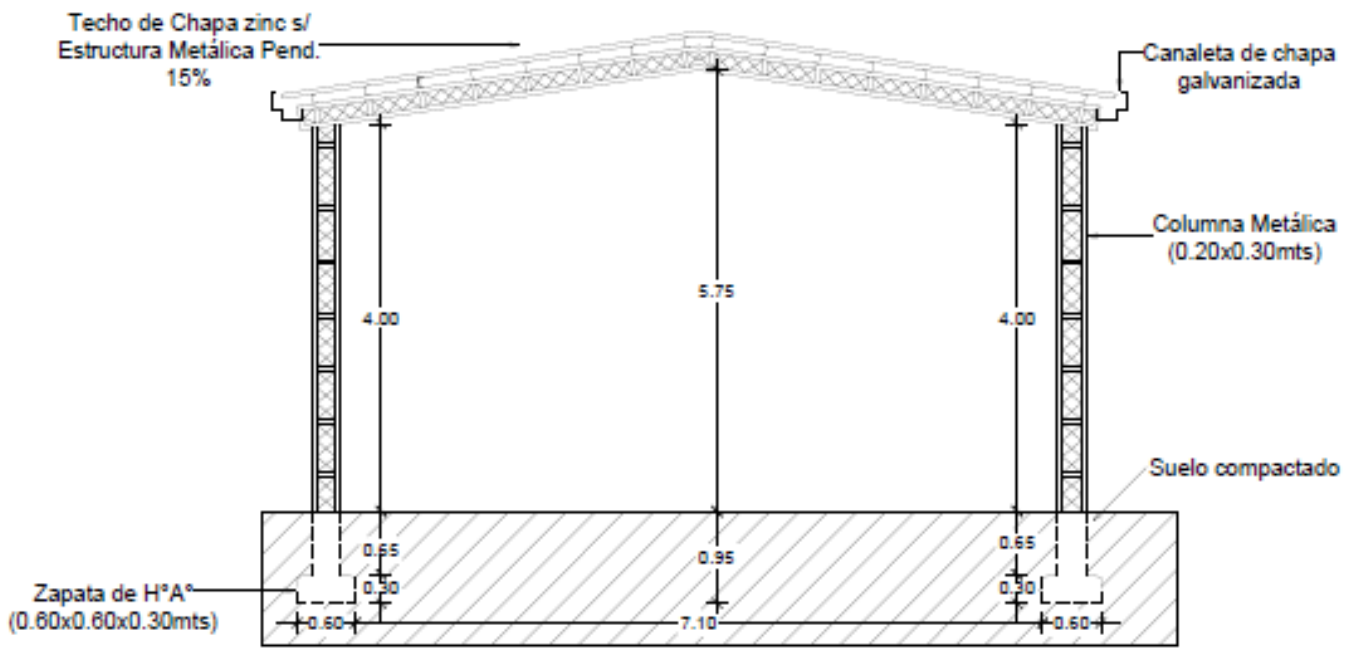
SECCIÓN TRANSVERSAL A-A'' ESC.:..... 1/75
