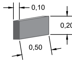
DETALLE DE CORDON ESCONDIDO DE H'A (10X50X20)
