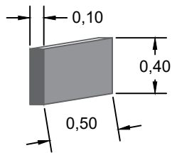
DETALLE DE CORDON NORMAL DE H'A (10X50X40)
