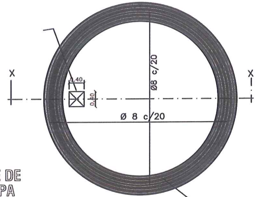
PLANTA POZO ABSORBENTE
