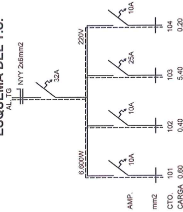
ESQUEMA DEL T.S.
