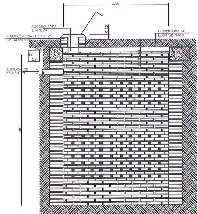
CORTE X-X
