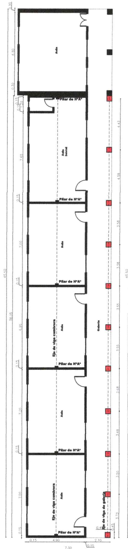
PLANTA BLOQUE 2 AULAS ESC. 1/100
