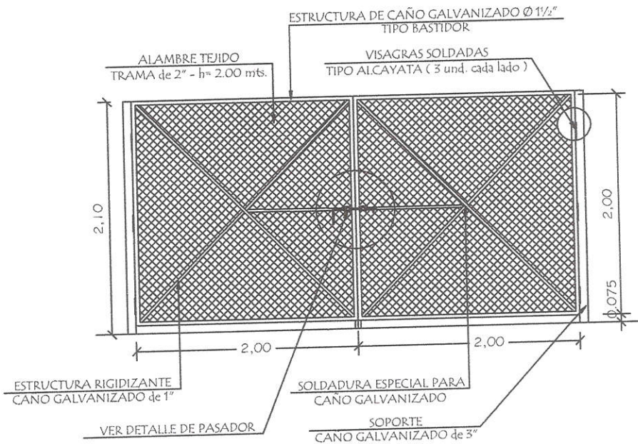
Portón de Acceso Vehicular de 4.00 x 2.00
