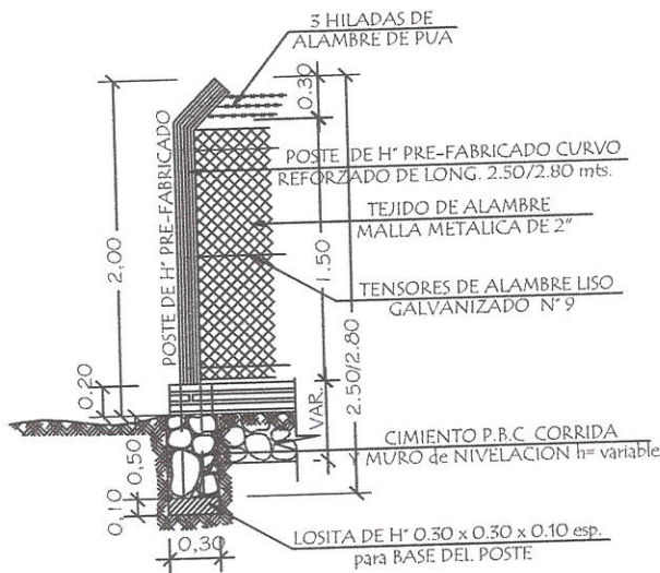
CERCADO PERIMETRAL
