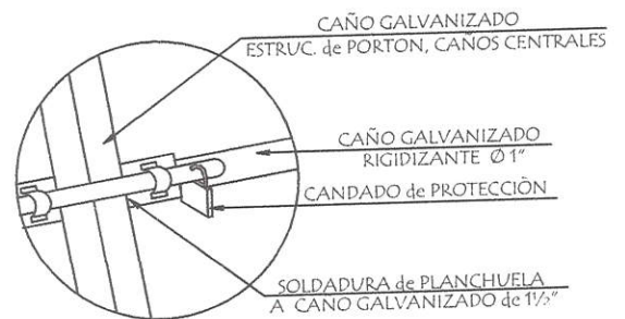
Detalle de Pasador
