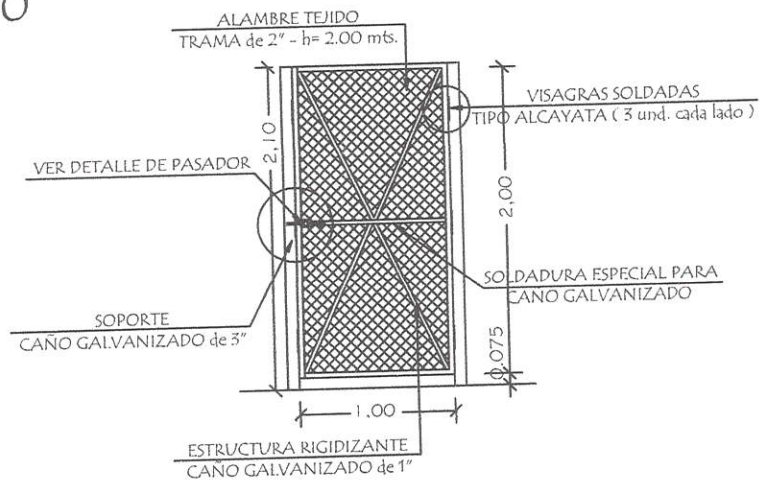
Portón de Acceso Peatonal de 1.00 x 2.00
