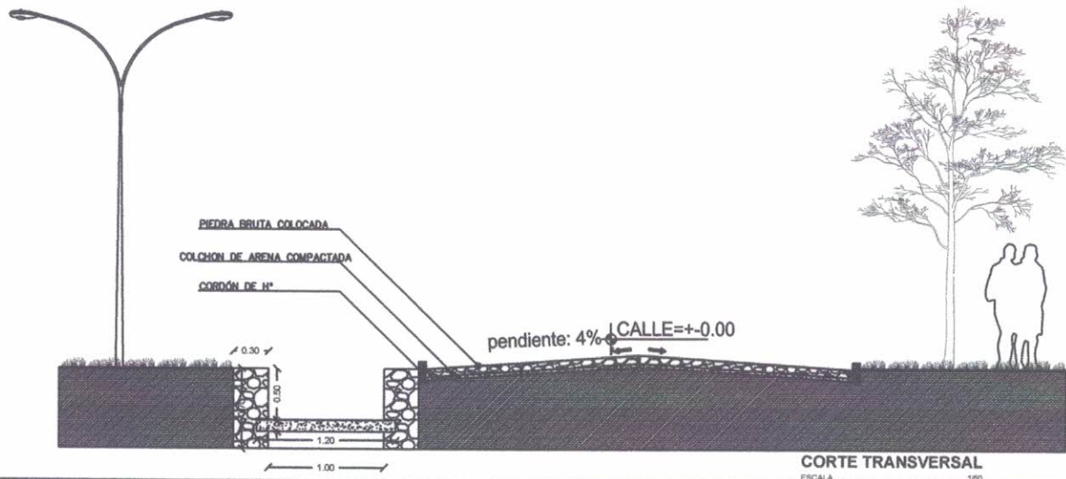
DETALLES DE CANALIZACIÓN
