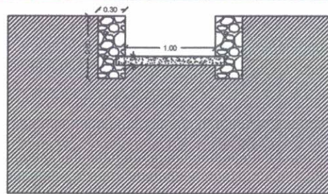
DETALLES DE CANALIZACIÓN
