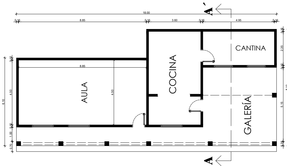
PLANTA ARQUITECTÓNICA ESCALA 1 100
