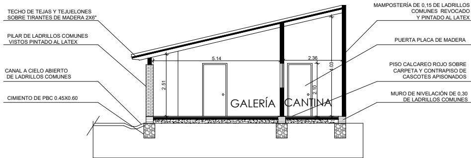
CORTE TRANSVERSAL A-A' ESCALA 1 100
