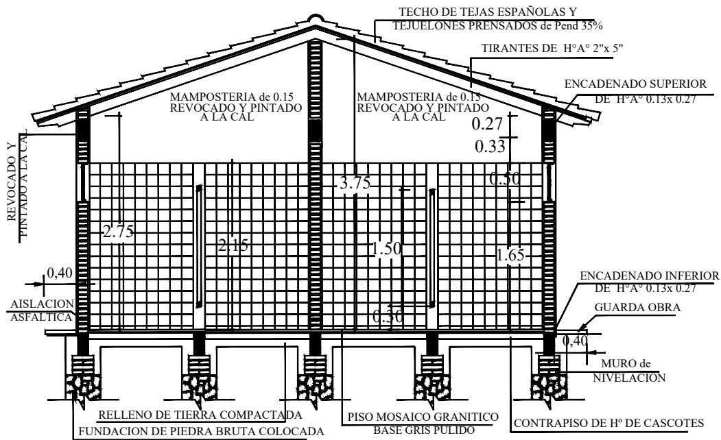
CORTE A-A'
