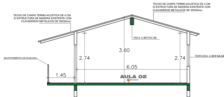
CORTE A-A PROYECTADO
