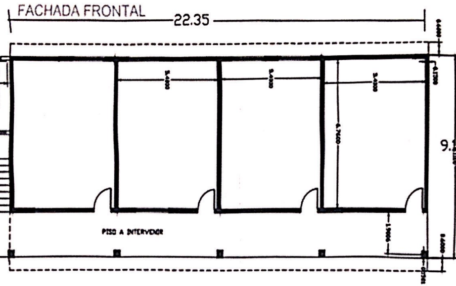
PLANTA BAJA
