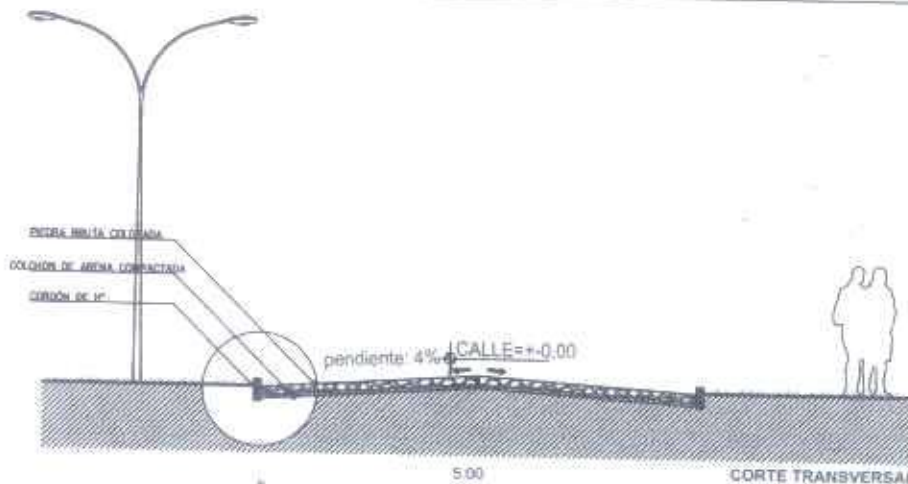
CORTE TRANSVERSAL
