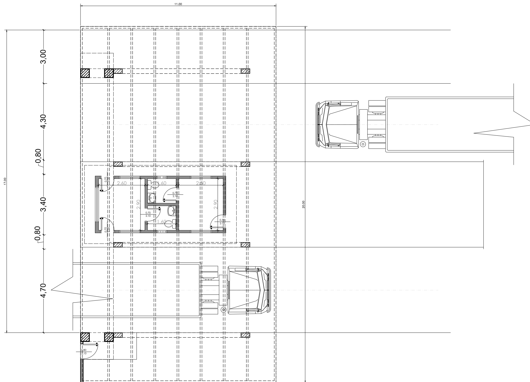
PLANTA PÓRTICO ESCALA 1/100
