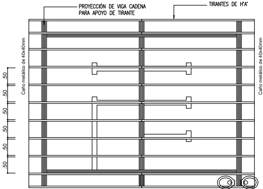
PLANTA DE TECHO SIN ESCALA
