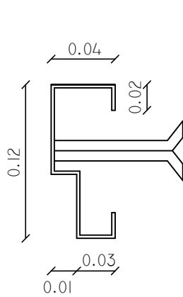
DETALLE DE MARCO
