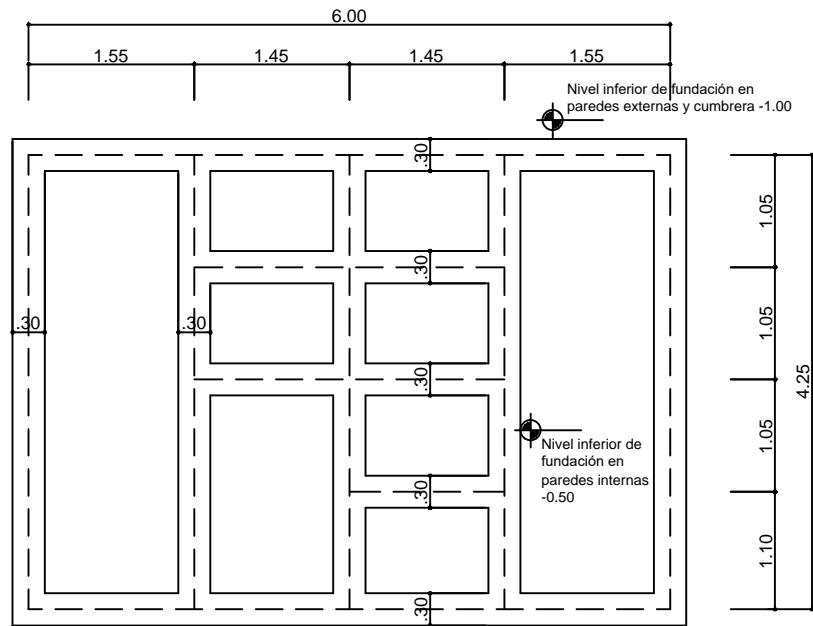
PLANTA DE FUNDACION SIN ESCALA
