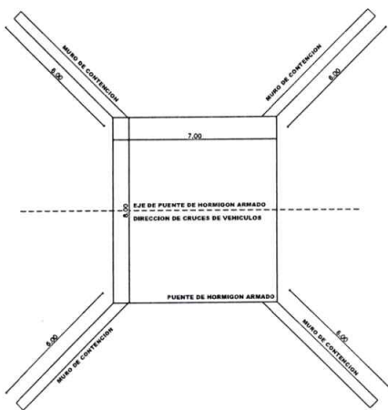
PLANO DE PUENTE DE H°A° ESC 1/50
