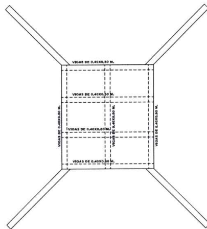
PLANO DE ENCOFRADO DE PUENTE DE H°A° ESC 1/50
