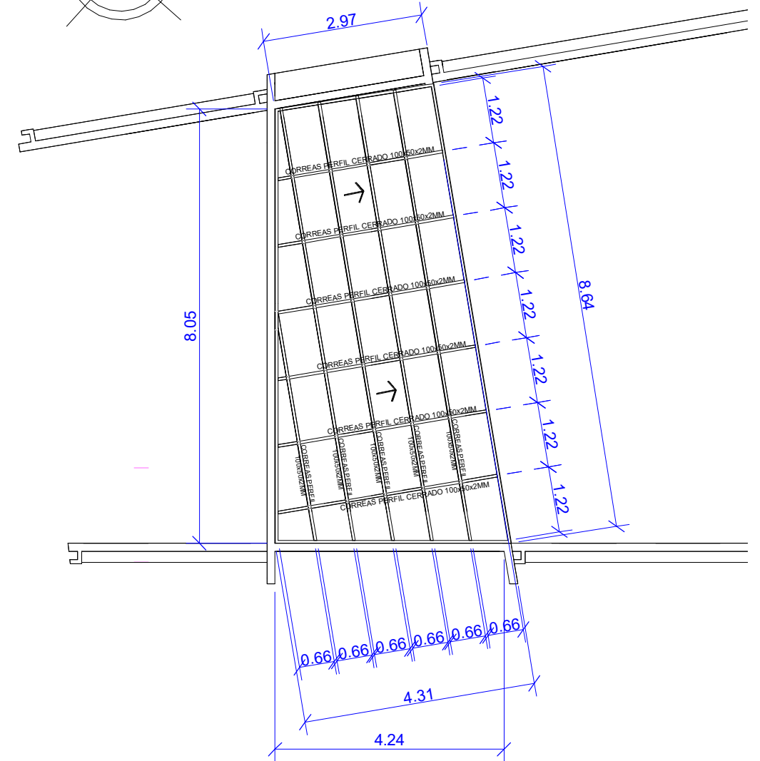
PLANTA DE ESTRUCTURA DE TECHO POLICARBONATO ESC:1.100
