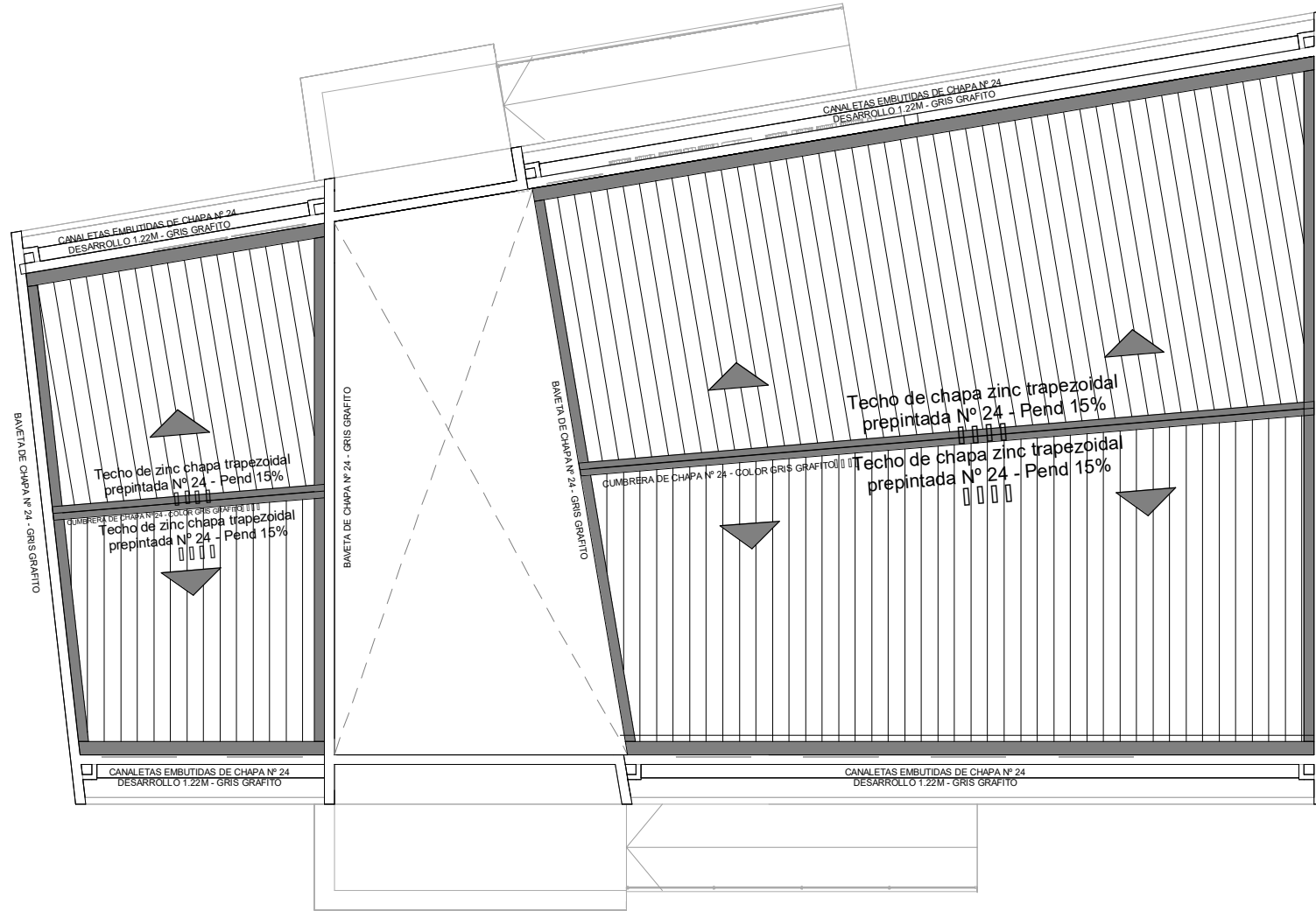
PLANTA DE DE TECHO ESC:1.100
