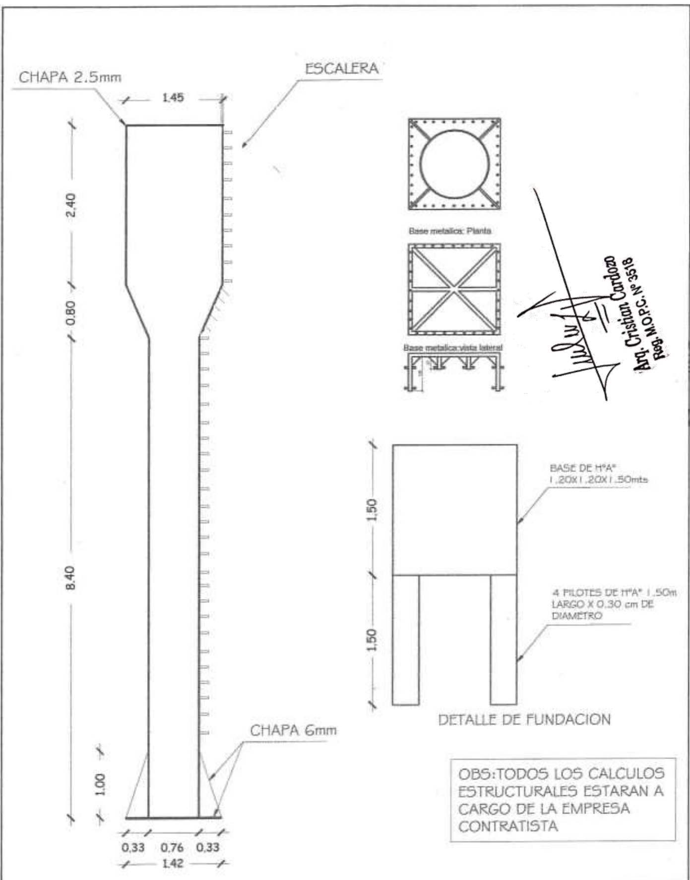
DETALLES DEL TANQUE DE 15.000 LTS.
