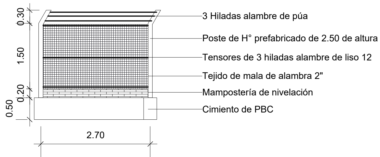
DETALLE DEL CERCADO EN LATERALES Y LA PARTE POSTERIOR
