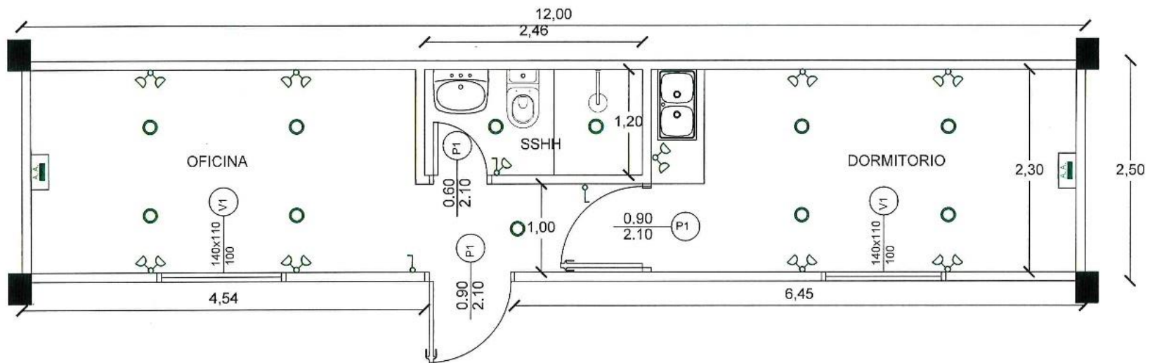
PLANTA - CONTENEDORES DE 40'
