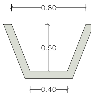
DETALLE DE CANAL ESCALA 1:50
