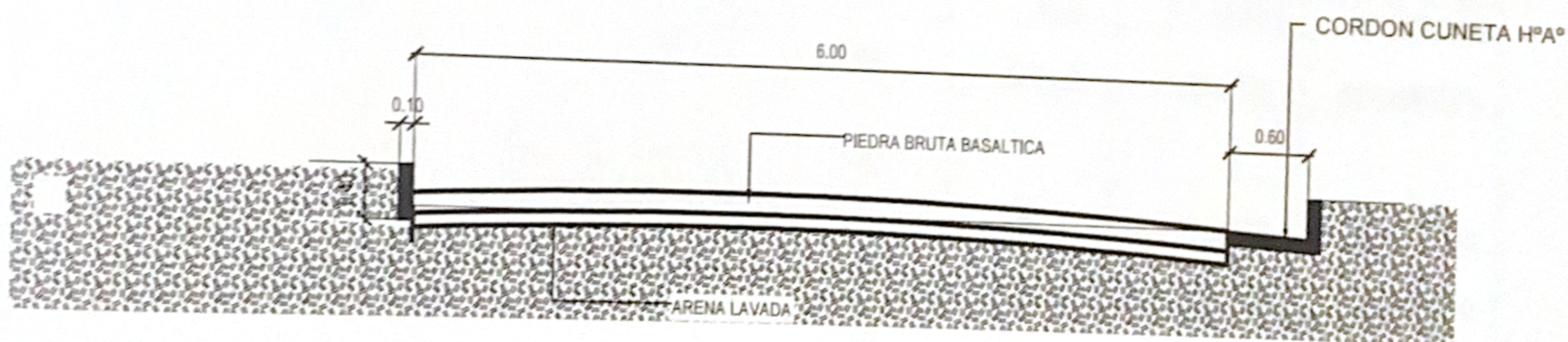
CORTE TRANSVERSAL
