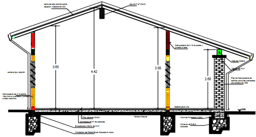
CORTE A - A EXISTENTE
