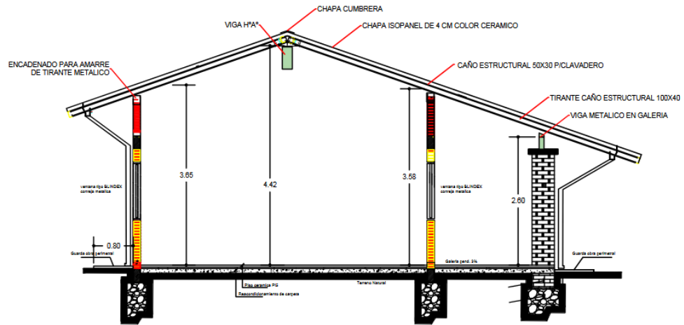
CORTE A - A PROYECTADO
