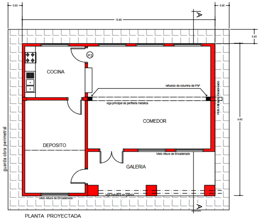
PLANTA PROYECTADA
