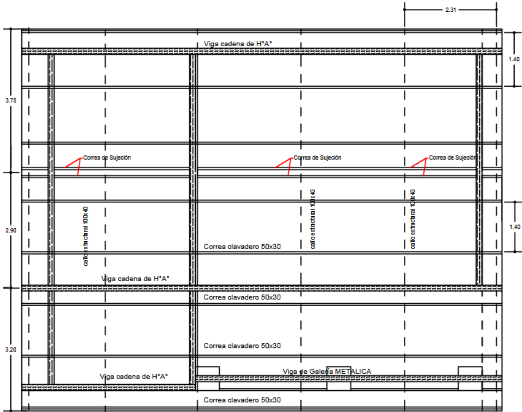
PLANTA DE TECHO PROYECTADA
