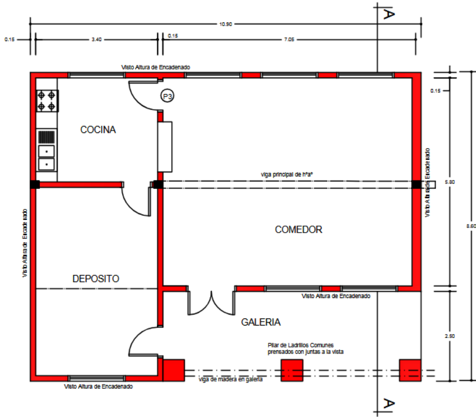
PLANTA EXISTENTE
