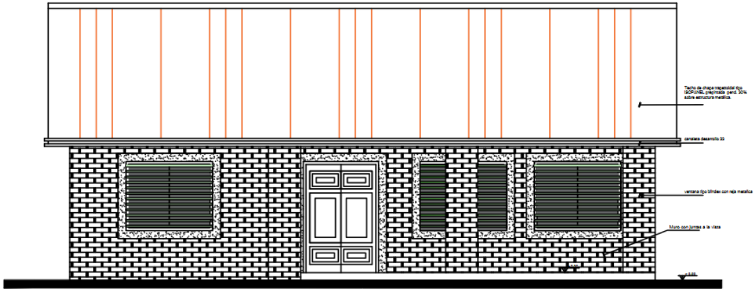
FACHADA FRONTAL PROYECTADA
