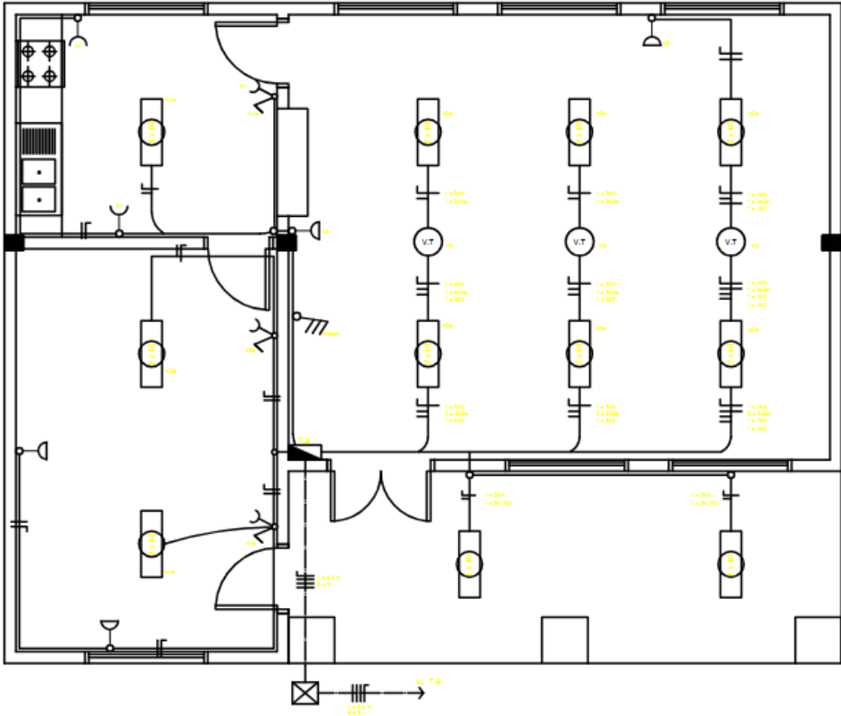
PLANTA INSTALACION ELECTRICA PROYECTADA
