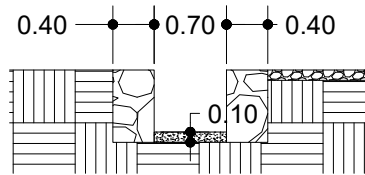
CANAL A CONSTRUIR
