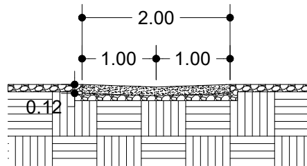
BADÉN DE HORMIGÓN ARMADO
