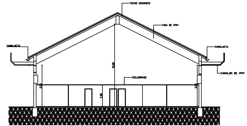
CORTE AA'
