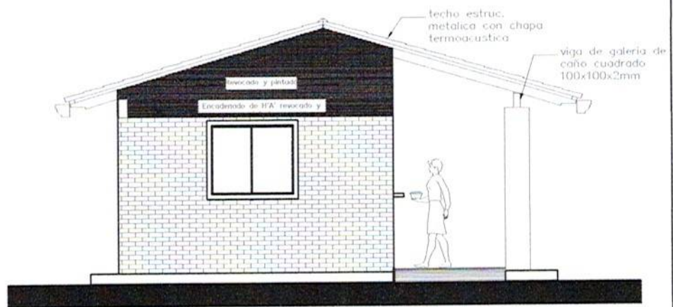
FACHADA LATERAL
