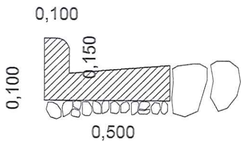
Detalle Cordón Cuneta. Esc.: 1:20
