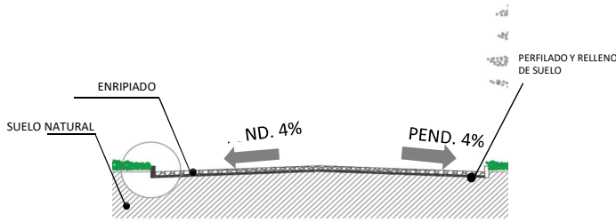
CORTE TRANSVERSAL DE LA CALLE S/E
