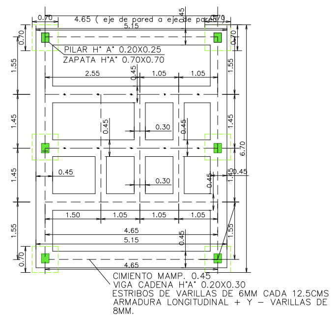
PLANTA DE CIMENTACION ESCALA.....1:100
