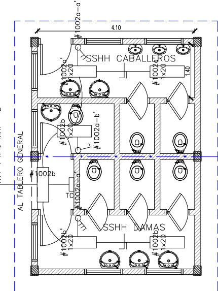
INSTALACION ELECTRICA ESCALA.....1:100
