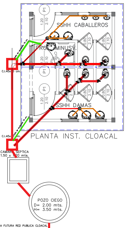
PLANTA ACOTADA ESCALA.....1:100
