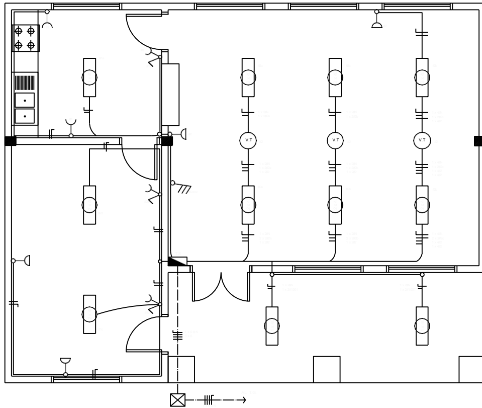
PLANTA INSTALACION ELECTRICA
