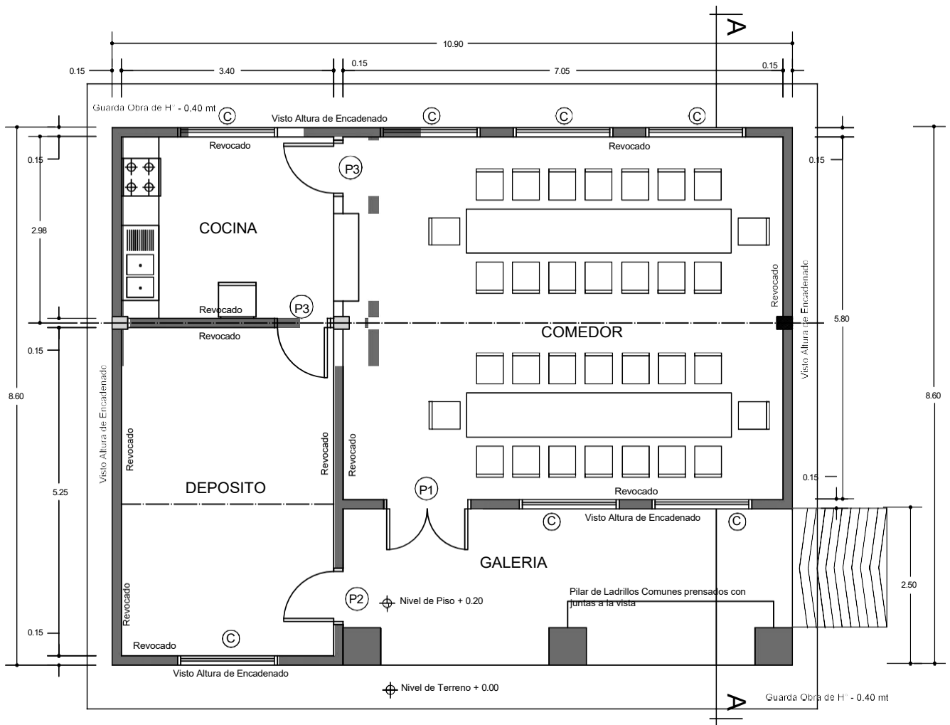
PLANTA ARQUITECTONICA
