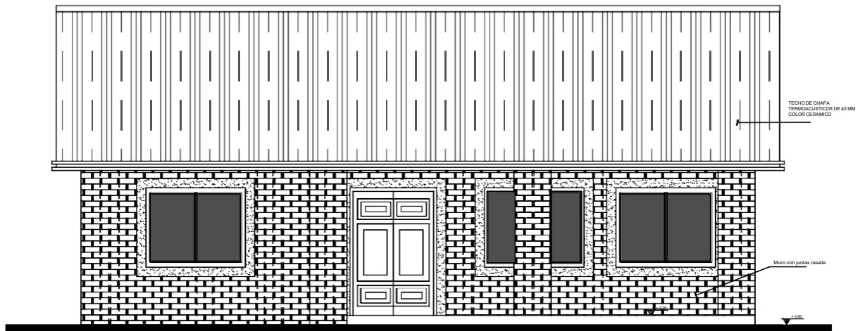
FACHADA FRONTAL
