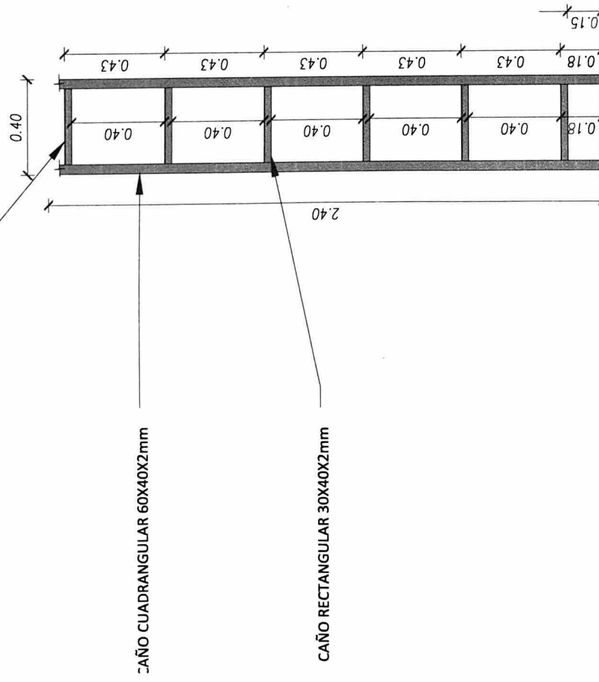
Esteriería metálica fachada lateral
