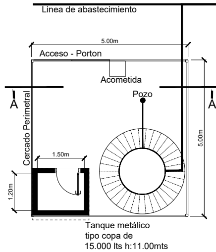
Planta Acotada
