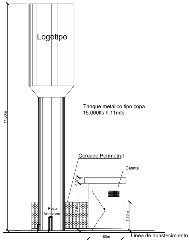
Corte AA'
