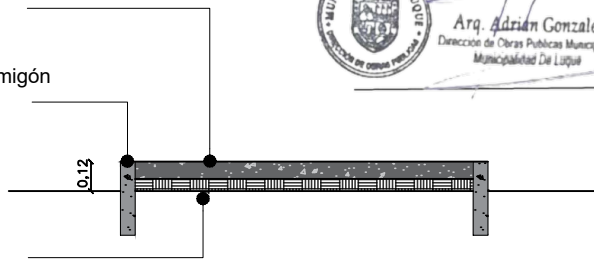
DETALLE CAMINERO HORMIGÓN
