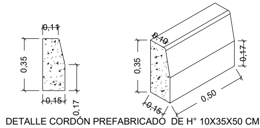
DETALLE CORDÓN PREFABRICADO DE H° 10X35X50 CM
