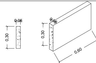
CORDÓN PREFABRICADO DE H° 6X30X60 CM
