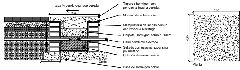
DETALLE REGISTRO ELÉCTRICO
