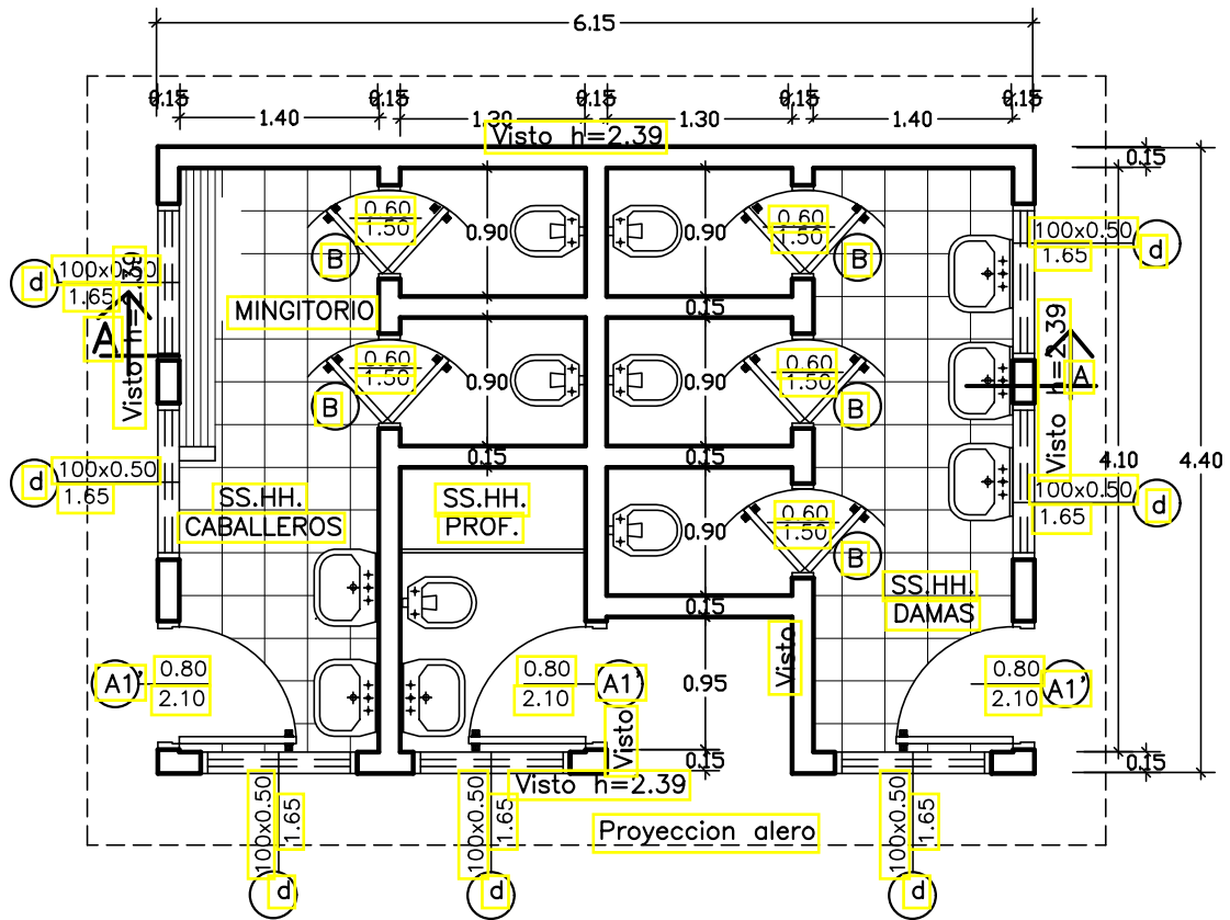
Planta constructiva esc. 1:50
