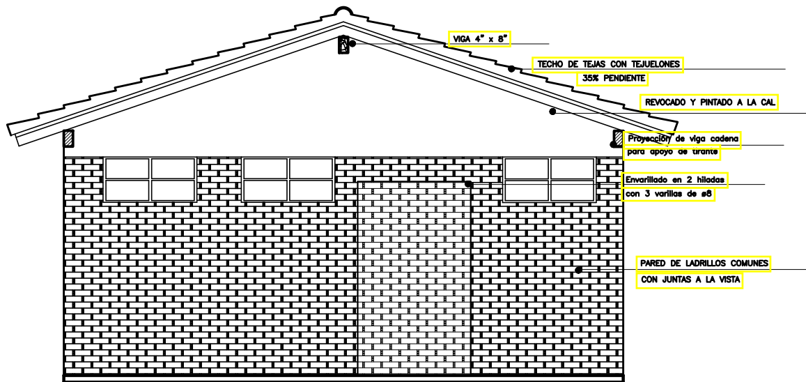
Fachada esc. — 1:50
