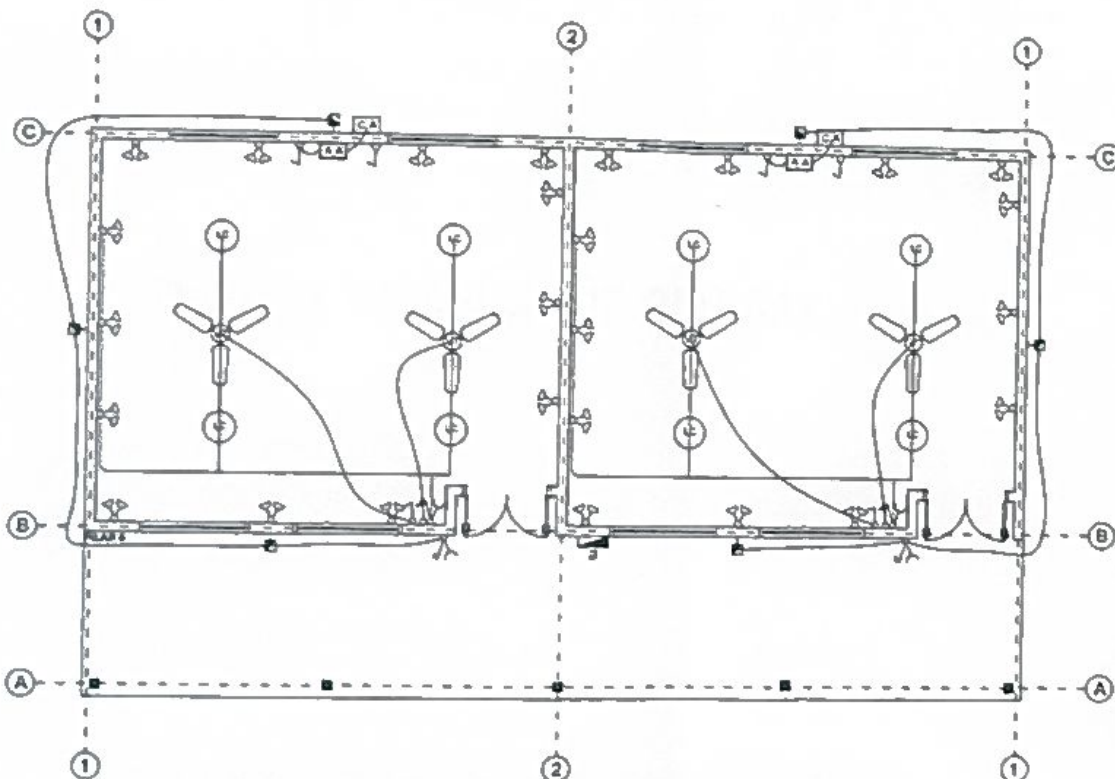
PLANTA DE INSTALACIÓN ELÉCTRICA
