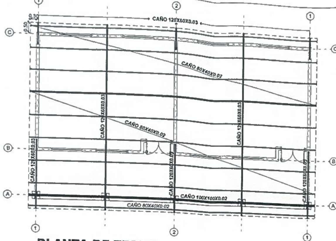
PLANTA DE TECHO
