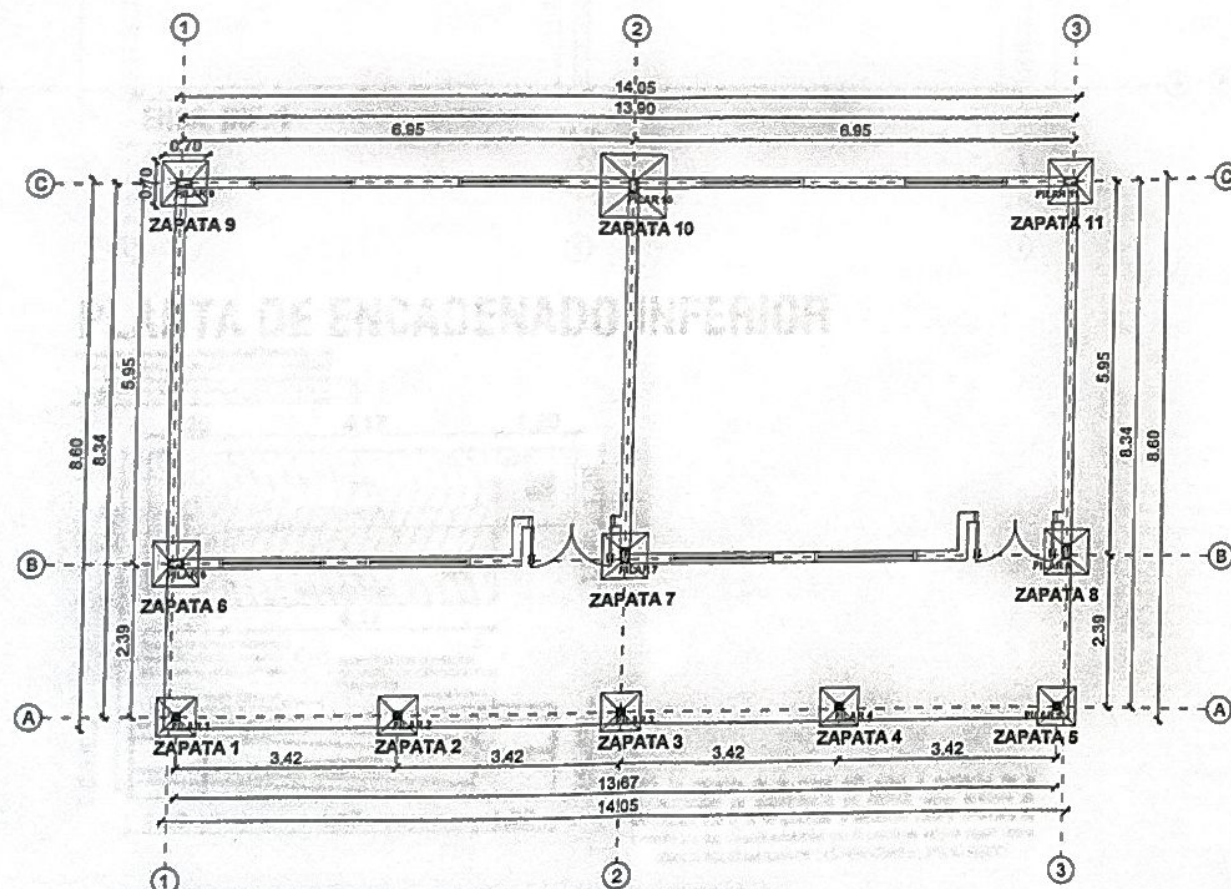
PLANTA DE PILARES Y ZAPATAS
