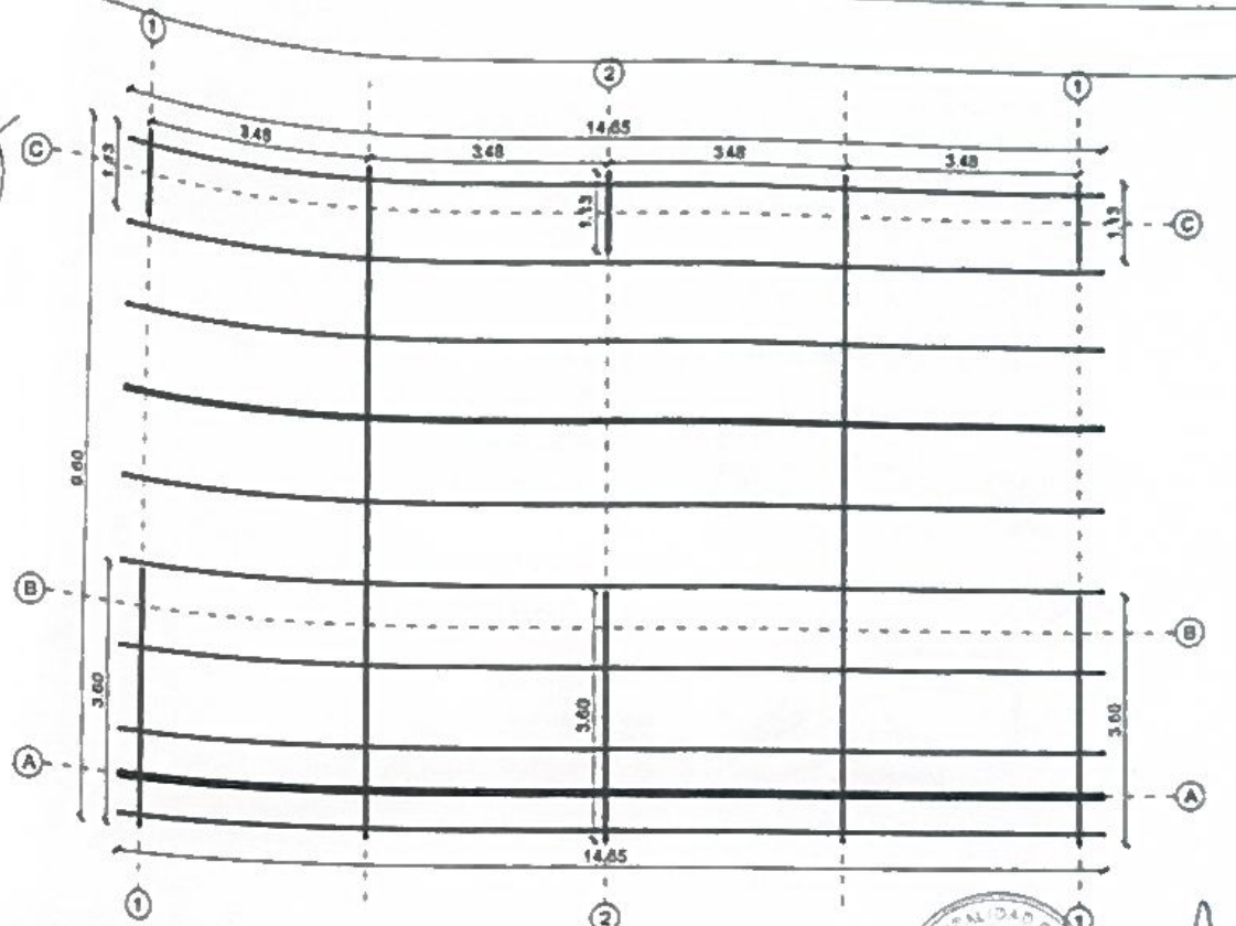
PLANTA DE ESTRUCTURA METÁLICA DE TECHO
