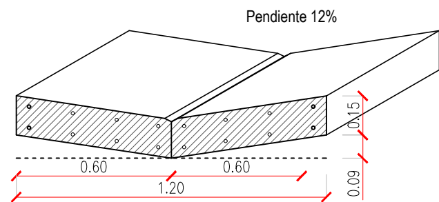
DETALLE DE BADÉN DE H°A° Esc.:_____1:20
