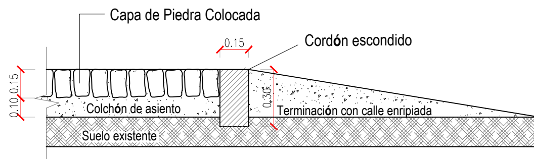
DETALLE DE CORDÓN ESCONDIDO DE H° Esc.: 1:20
