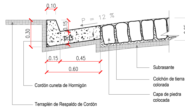
CORTE CORDÓN CUNETA DE H° Esc.: _____ 1:20
