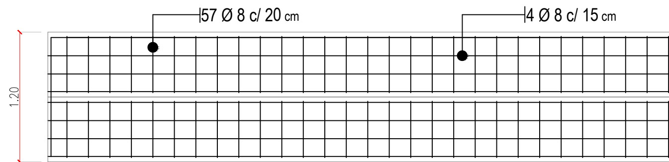
BADÉN DE HORMIGÓN ARMADO Esc.: _____ 1:35
