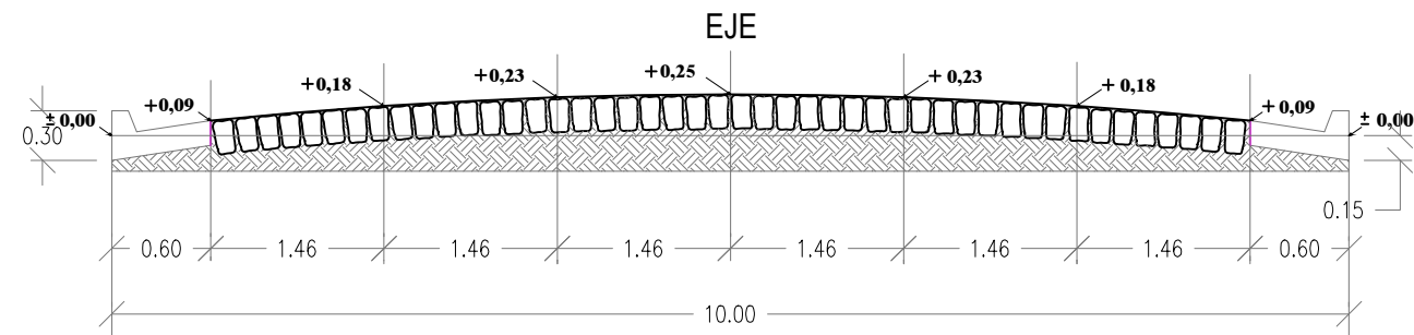
CORTE TRANSVERSAL TIPO Esc.: _____ 1:50
