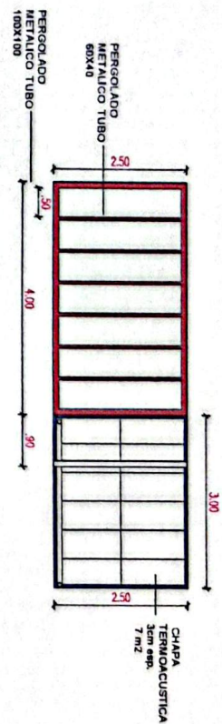
CASILLAS COMERCIALES PLANTA CUBIERTA VISTA SUPERIOR
