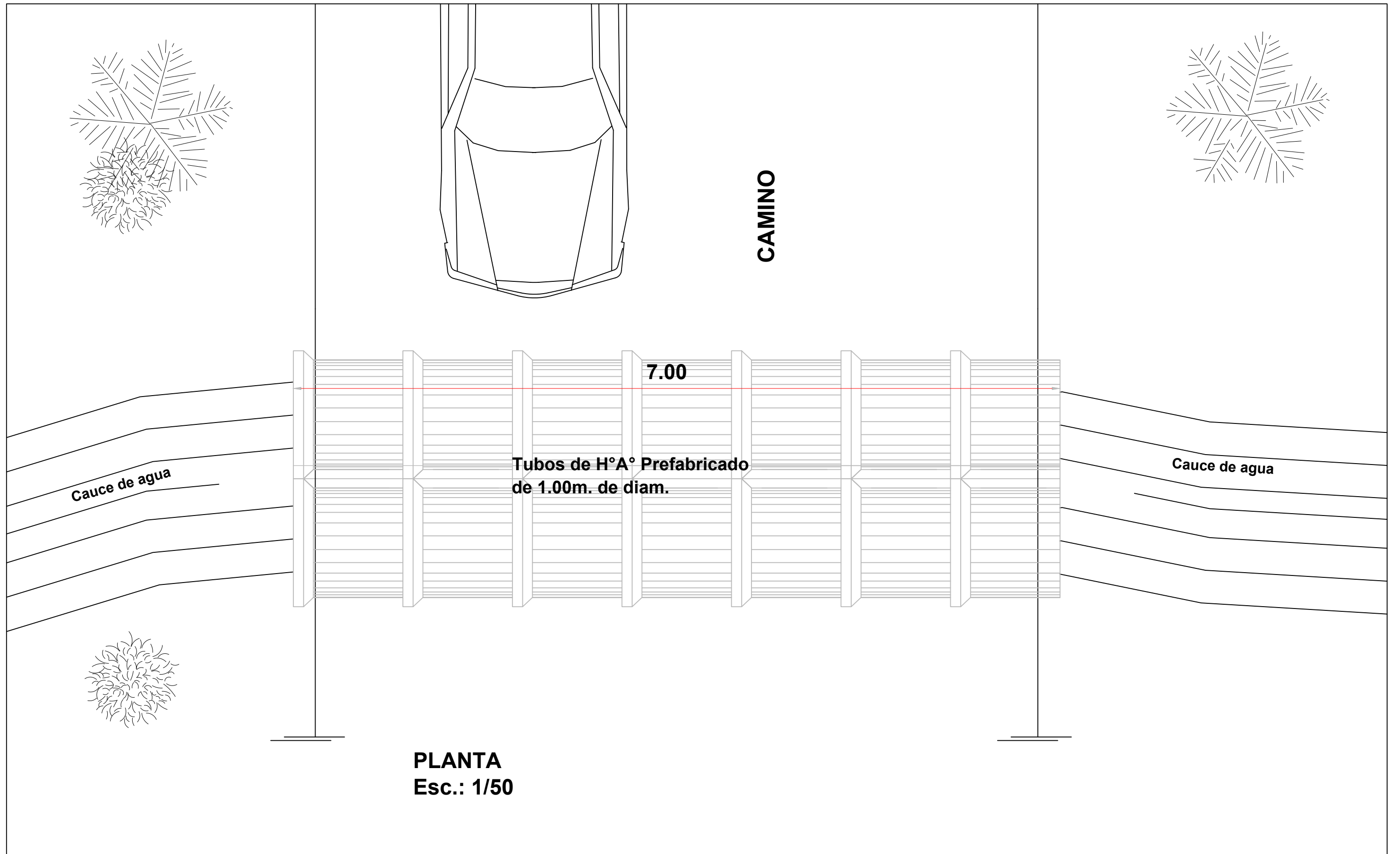
PLANTA - ALCANTARILLADO Esc.: 1/50
