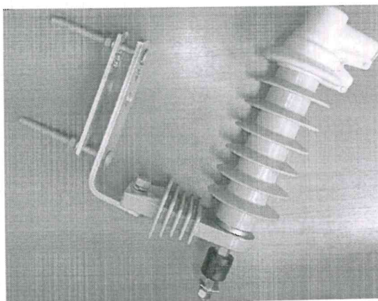
Vista del Descargador con sus accesorios de sujeción y la cobertura aislante de protección
