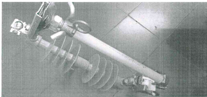
Vista de perfil del Seccionador Fusible Unipolar con el Portafusibles
