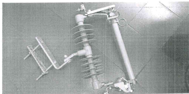
Vista general del Seccionador Fusible Unipolar con el Portafusibles y su correspondiente soporte de fijación
